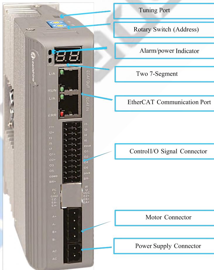
EM3E-A882
